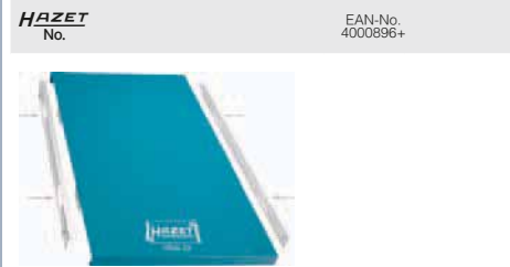
Zusatz-Einlegeboden für Werkbank 179 W Für den flexiblen Einbau im rechten Regalteil auf der Vorderseite Belastbarkeit 15 kg 179 W-23 150311
